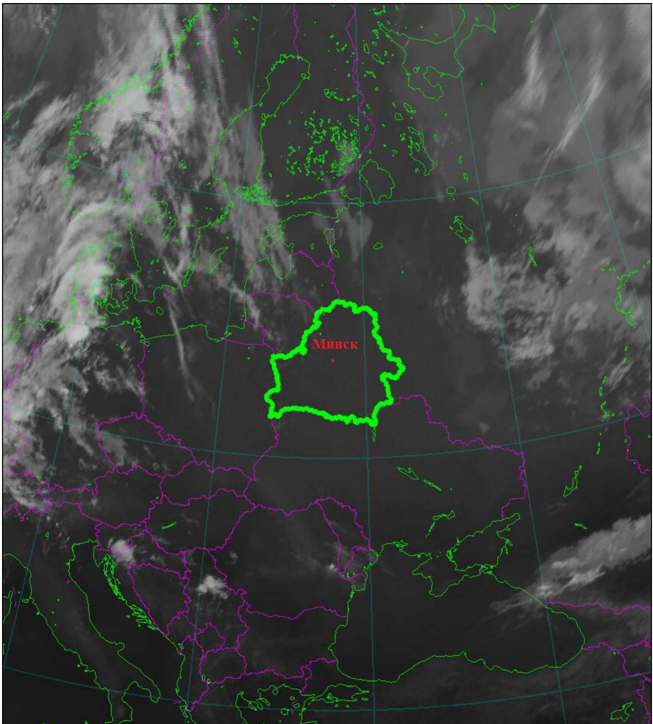
Снимок облачности с искусственного спутника Земли (ИСЗ) на 8 часов 00 минут 15 августа 2024 г.
